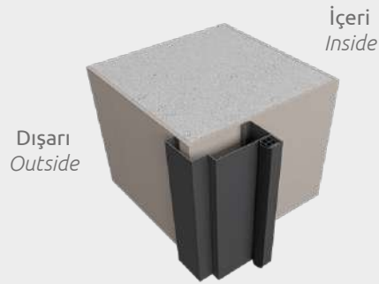
Dışardan Geçme Dışa Açılır Kasa (Rus Tipi) External Mounted Fixed Frame-Opening Outwards (Russian Type)
