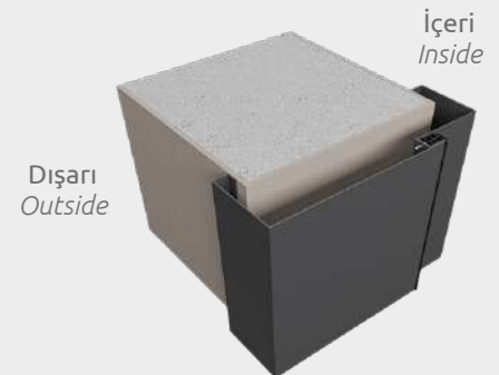
Fitol Altından Vidalamalı SABİT Kasa Hidden Screwed Fixed Frame
