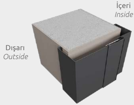
Fitil Altı Vidalamalı Ayarlı Kasa Hidden Screwed Adjustable Frame
