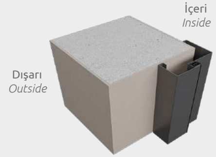
İçerden Geçme Kasa (Açık Tip) Internal Mounted Fixed Frame (Standard Type)
