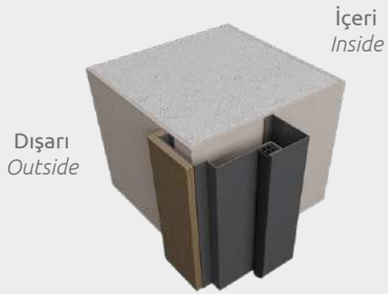
Dışardan Geçme Dışa Açılır Kaplamalı Kasa (Rus Tipi) External Mounted Fixed Covered Frame-Opening Outwards (Russian Type)
